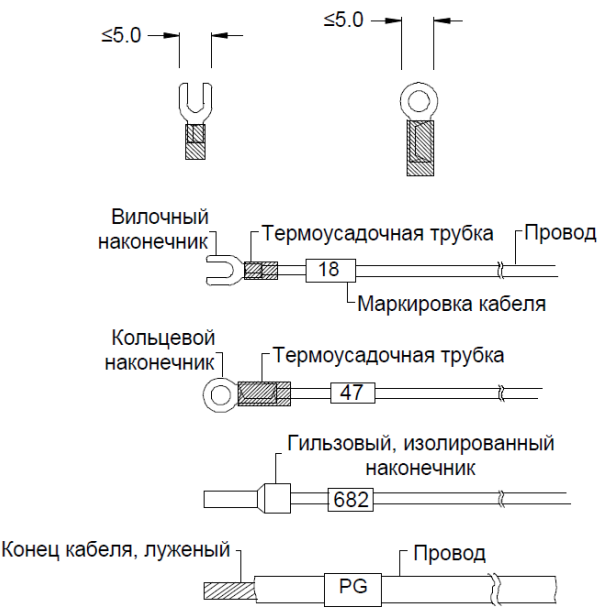
Рис. 5.4 Рекомендованный способ подготовки проводов
