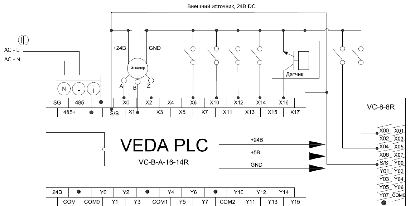
Рис. 3.1.2 Пример подключения входов
