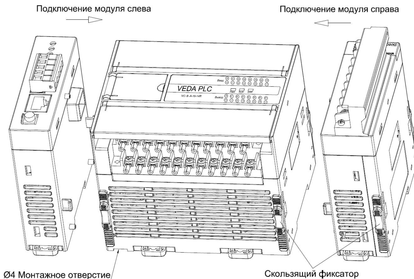
Рис. 5.2.2 Подключение модулей расширения
