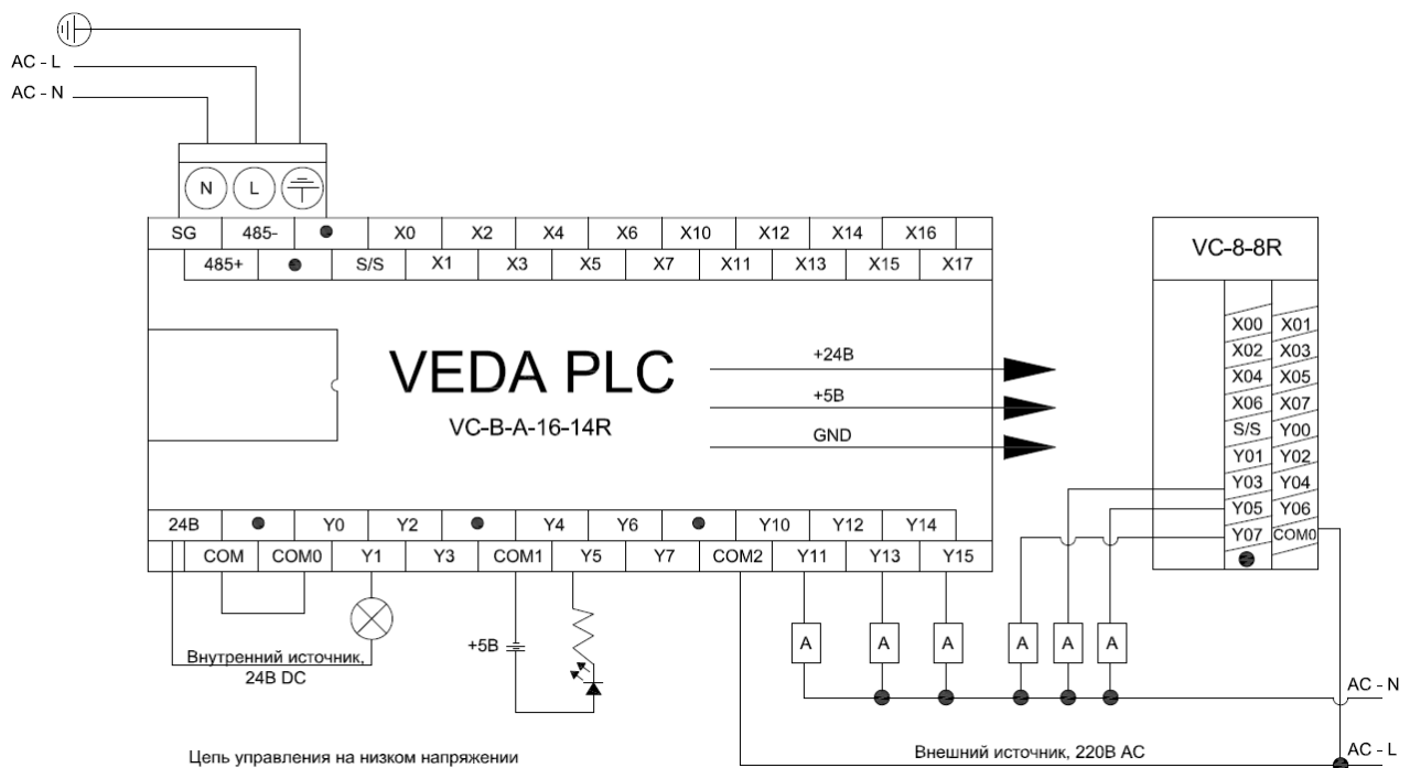
Рис. 3.2 Пример подключения выходов
