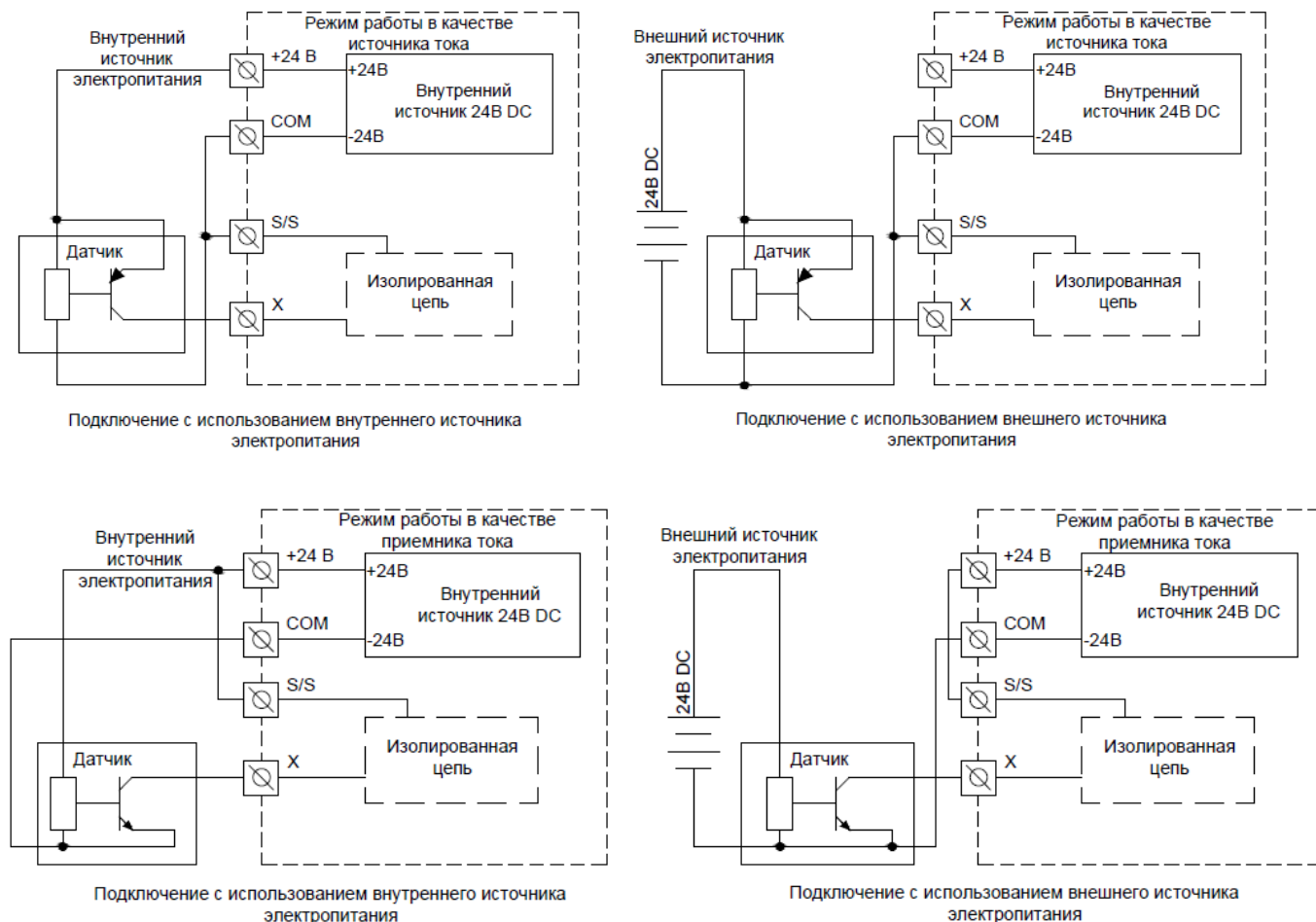
Рис. 3.1.1 Пример подключения входных сигналов
