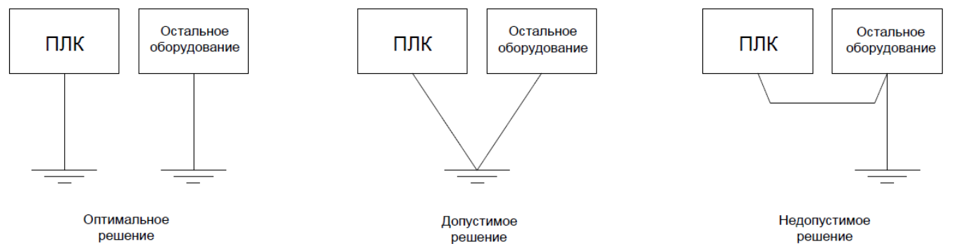
Рис. 5.3 Заземление ПЛК
